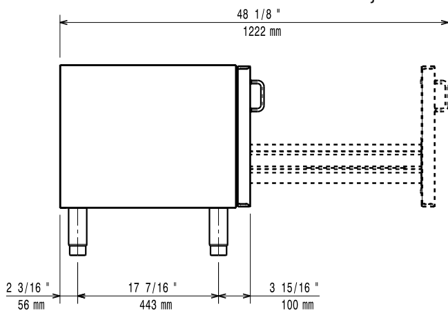
Boven aanzicht
